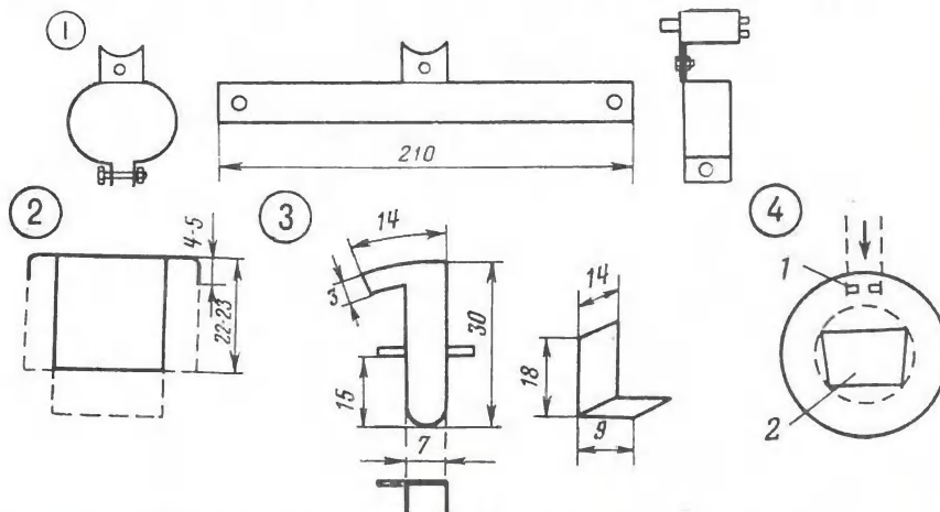
Рис. 1. Держатель.
