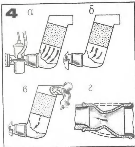
4. вследствие уменьшения количества воздуха, поступающего в карбюратор: а — неисправен воздухоочиститель; б — засорен пылью фильтр; в — в воздухоочистителе попали посторонние предметы; г — деформирован соединительный патрубков воздухоочистителя;
