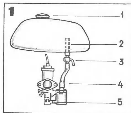
1. вследствие уменьшения количества топлива из-за засорения: 1 — отверстия в крышке бака; 2 — сетчатого фильтра; 3 — бензокраника; 4 — бензошланга; 5 — топливных каналов и жиклеров карбюратора;
