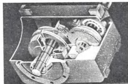
Общий вид экспериментальной бесступенчатой трансмиссии «Трансматик».
