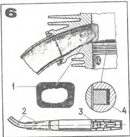
6. при отложении нагара: 1 — в выпускном окне; 2 — в выпускной трубе; 3 — в акустическом фильтре (вставке) глушителя; 4 — в канавках поршня (закосковывание колец).
