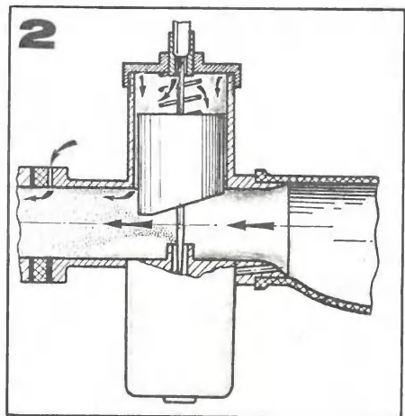
2. вследствие поступления лишнего («постороннего») воздуха через соединения карбюратора с патрубком, если повреждена прокладка;
